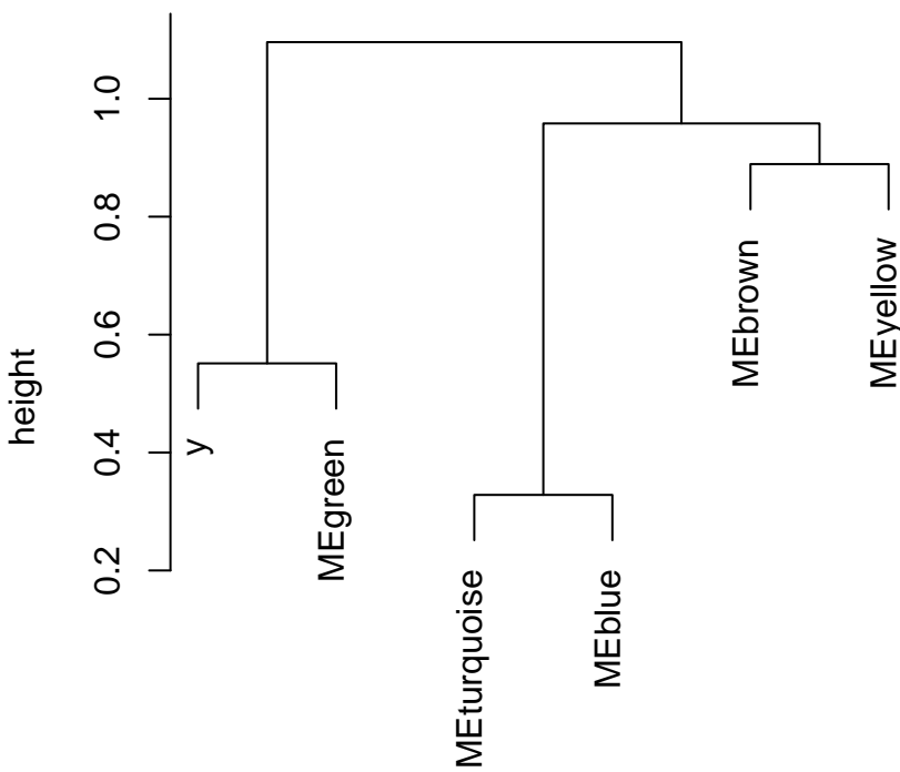
C. Module eigengene dendrogram
