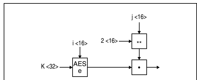
Figure 7-337. Compute XTS Parameter Using AES 256
