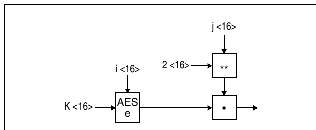
Figure 7-334. Compute XTS Parameter Using AES 128
