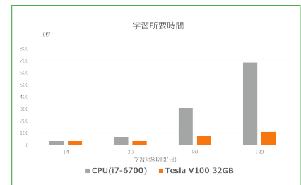
LSTMにおいて、CPUとGPUの学習所要時間を比較したグラフ。学習対象期間が180日の場合、GPUでは84%の時間削減になる
