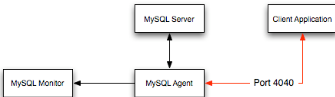
図9.3 MySQL Enterprise Monitor User Interface: Query Analyzer エージェント/モニタートポロジ
