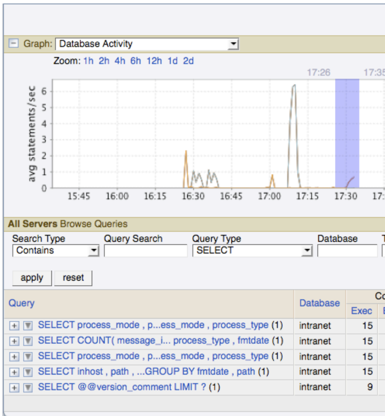
図9.7 MySQL Enterprise Monitor User Interface: 相関グラフ
