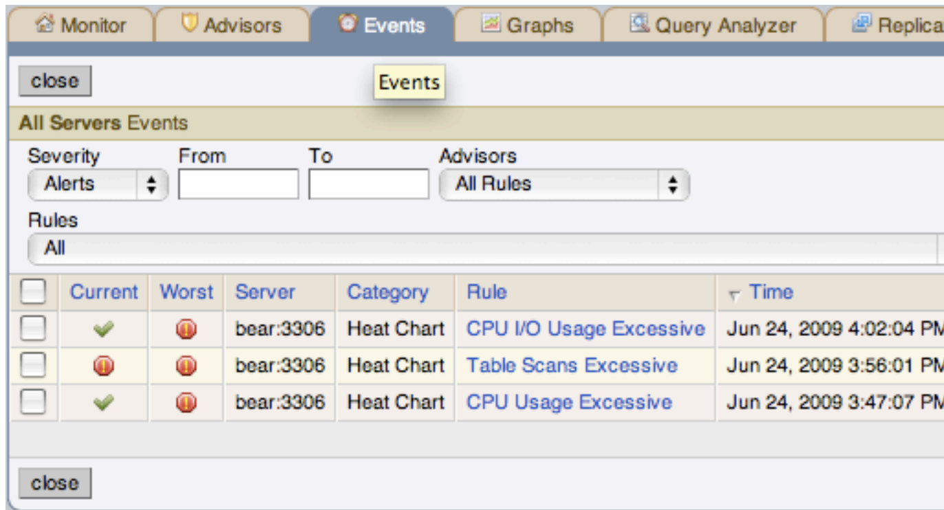
図7.1 MySQL Enterprise Monitor User Interface: イベント画面
