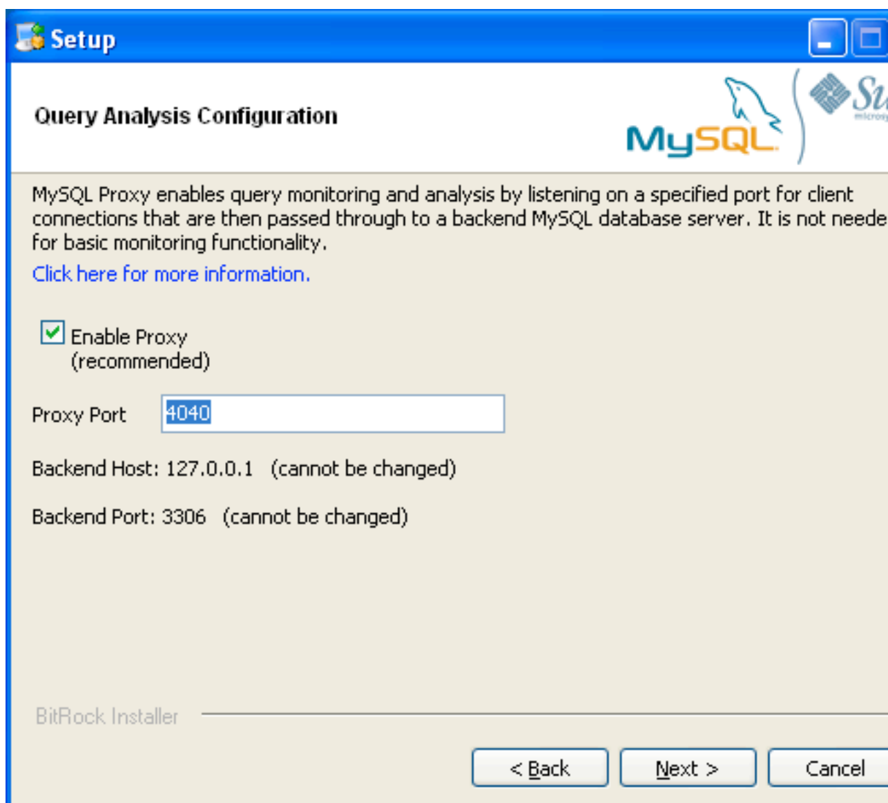
図2.15 MySQL Enterprise Monitor: Windows での Agent のインストール: Query Analyzer の設定
