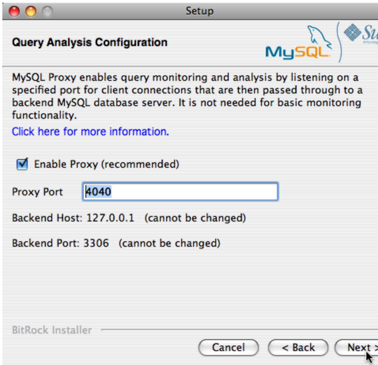
図2.21 MySQL Enterprise Monitor: Mac OS X での Agent のインストール: Query Analyzer の設定
